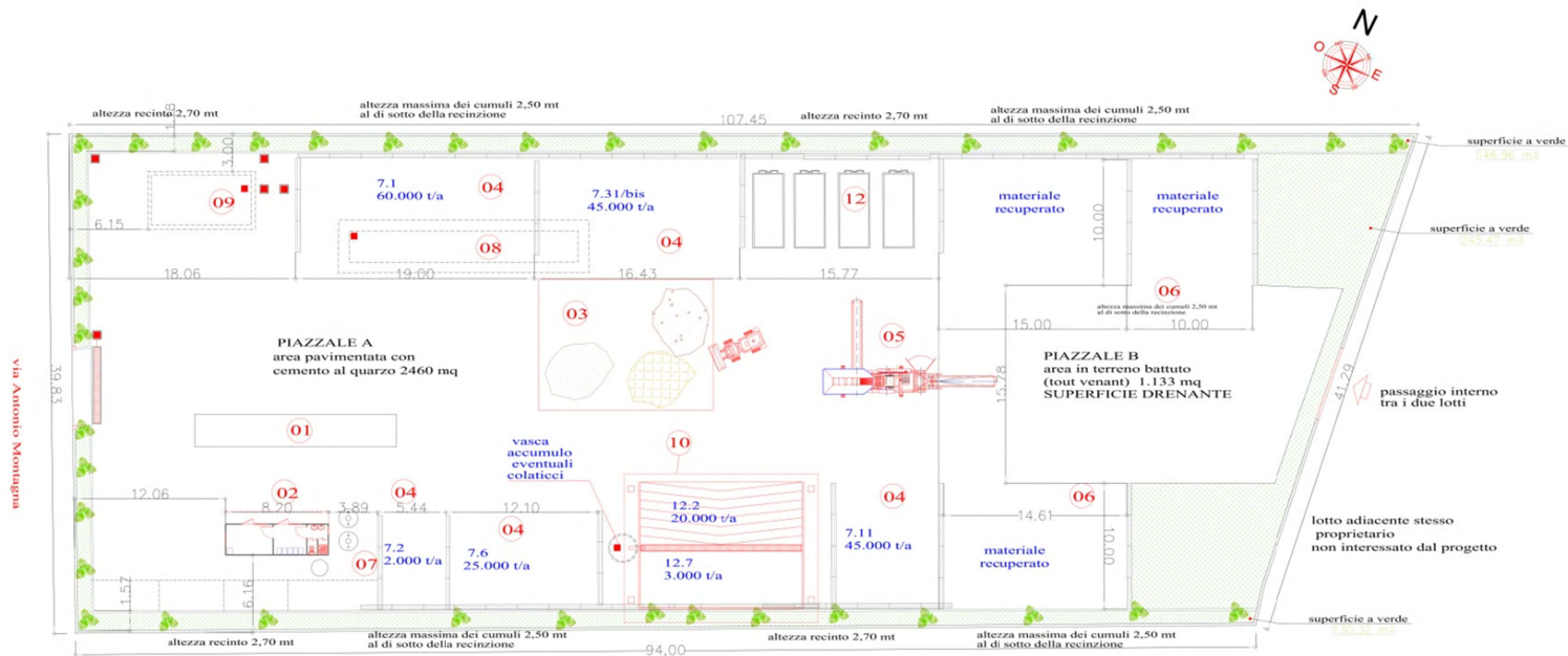
Planimetria Generale scala 1:200
